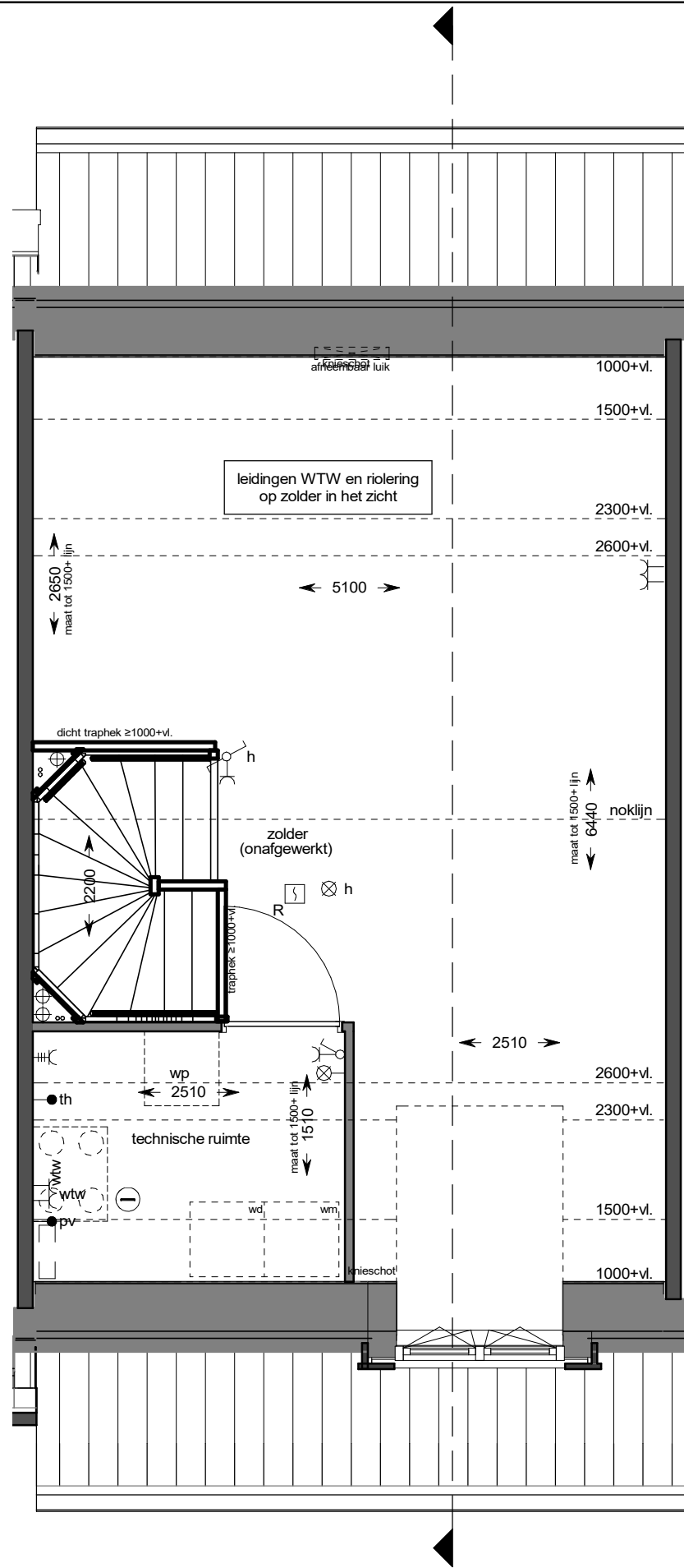
tweede verdieping
