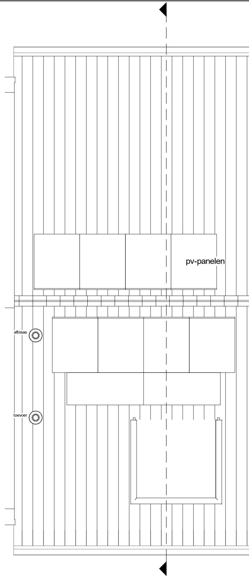
dakaanzicht
